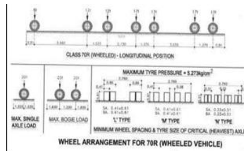
FIG 3. 70R WHEELED LOAD
