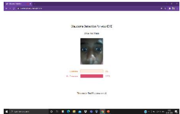
Fig 6. Web UI
