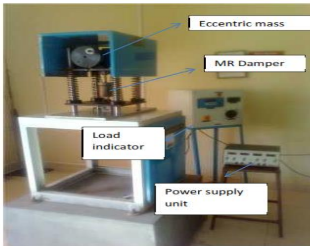
Fig. 4.1 MR Damper test rig.
