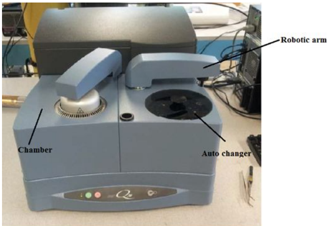
Fig. 4.5 DSC apparatus
