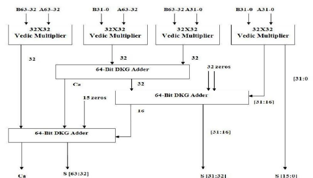
Fig 3: 64 \times 64 Vedic multiplier using 32 \times 32 Vedic multiplier
